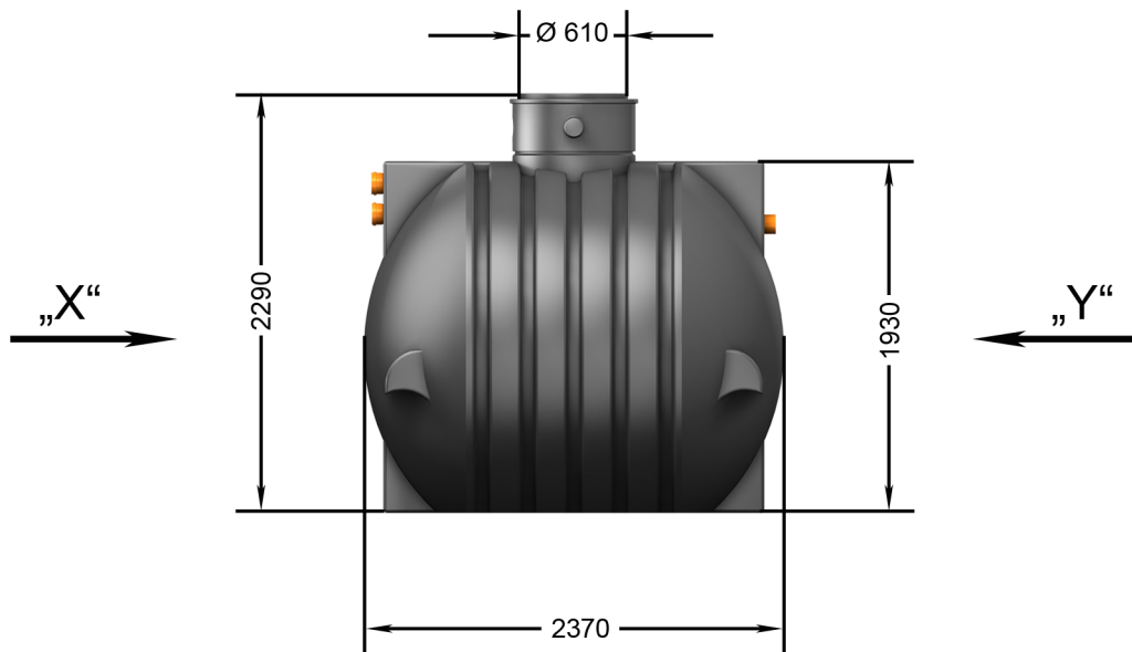
Ansicht „X“
